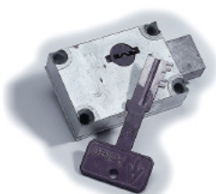
Cerradura de Detención con Llave Paracéntrica
