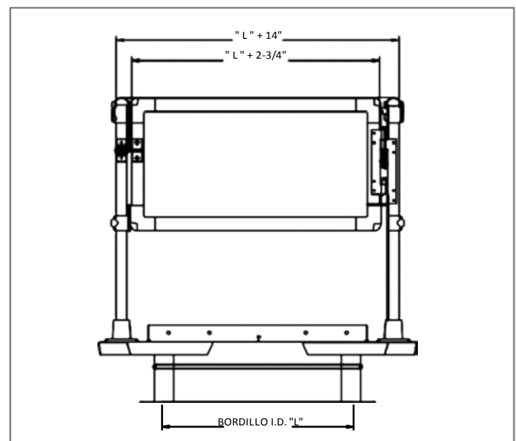
ESCOTILLA DE AZOTEA Y BARANDALES DE SEGURIDAD VISTA FRONTAL (CUBIERTA DE ESCOTILLA DE AZOTEA REMOVIDA PARA UNA MEJOR VISTA DEL SISTEMA DE BARANDAL)
